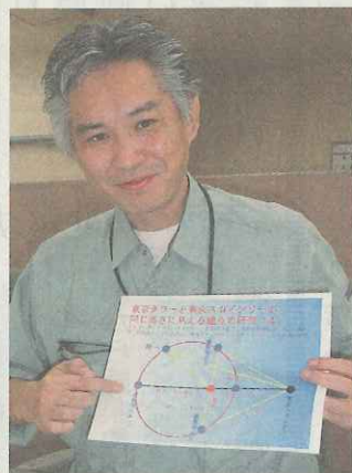
アポロニウスの円上で同じ高さに見えると話す三矢宏さん
